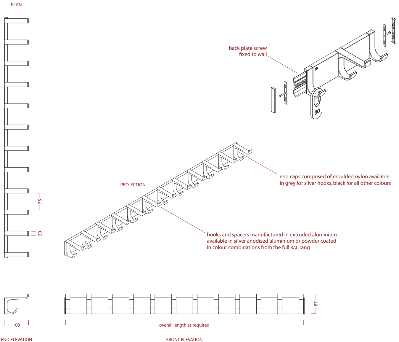
END ELEVATION
