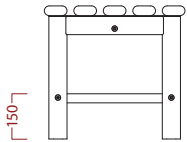
END ELEVATION
